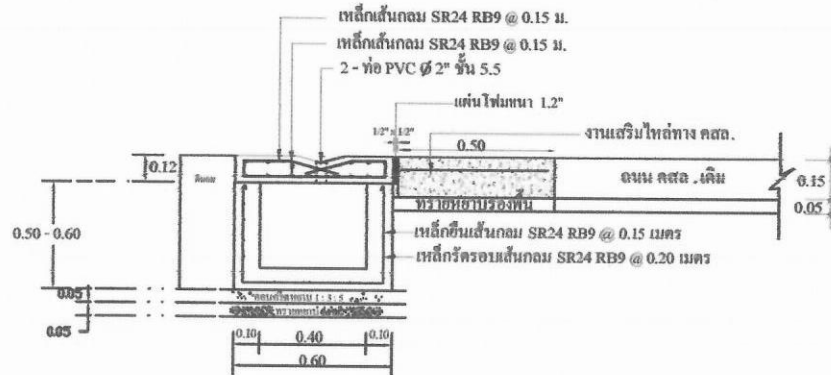
ขยาย รูปตัดตามขวาง
