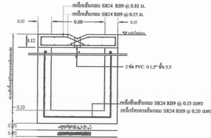
รูปตัดบ่อพักน้ำ คสล.
