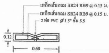
แปลนขยายฝ่าปิด คสล.
